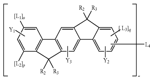
[Chem 3]
