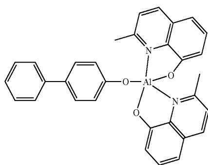
BAlq
